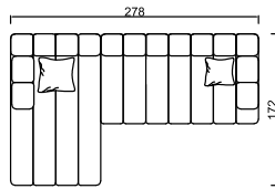
Corner / Köşe 172x278x72
